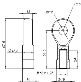
Шаровой шарнир ЛА50
