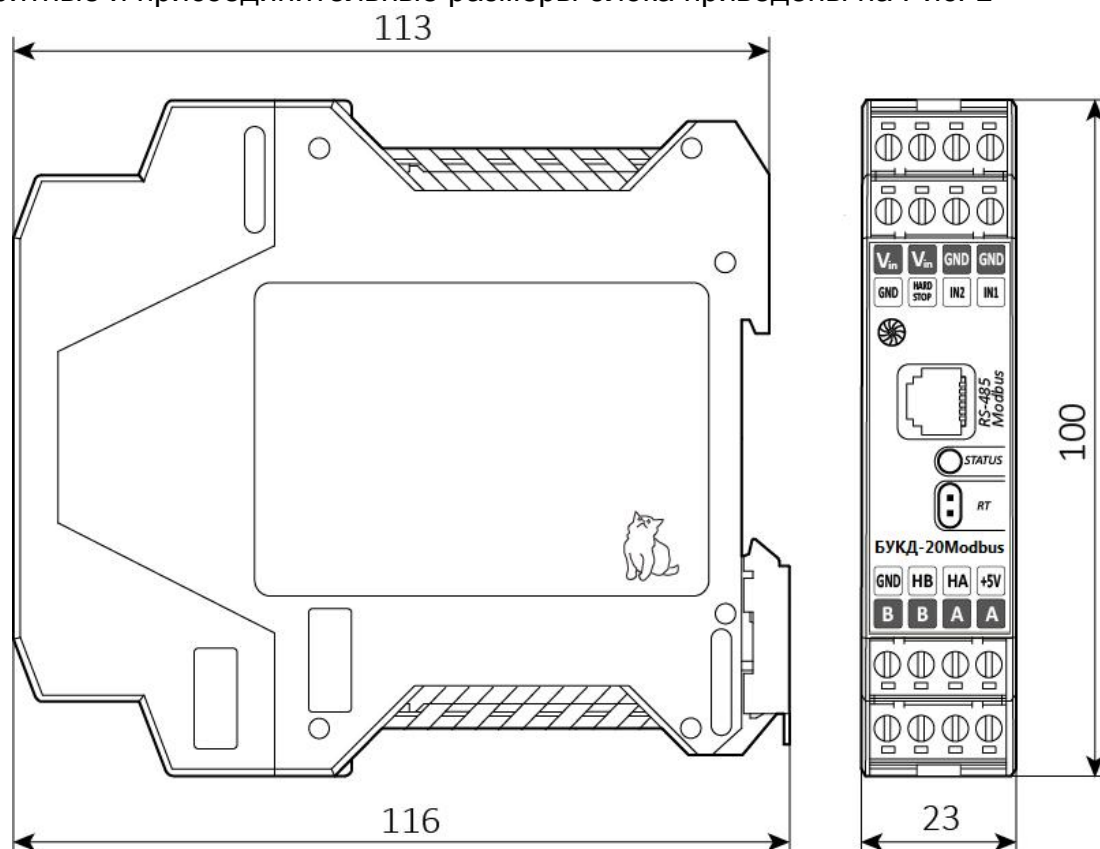
Рис.1. Габаритные и присоединительные размеры блока БУКД-20Modbus и БУКД-40Modbus
