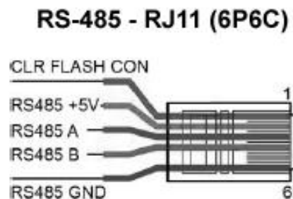
Рис. 4 – назначение контактов разъема RJ11 – RS-485 Modbus.
