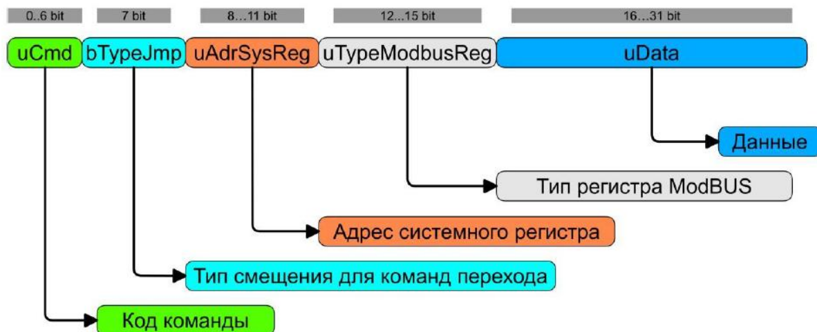
Рис.9 – структура инструкции пользовательской программы
