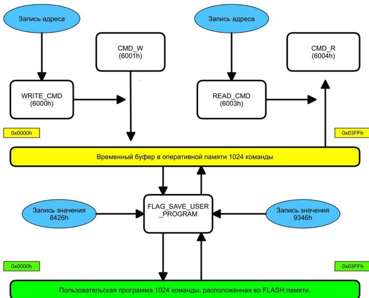
Рис.8. Блок-схема процедур чтения и записи пользовательской программы.
