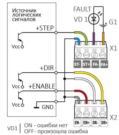
Рис. 2. – Подключение блока по схеме с общим катодом
