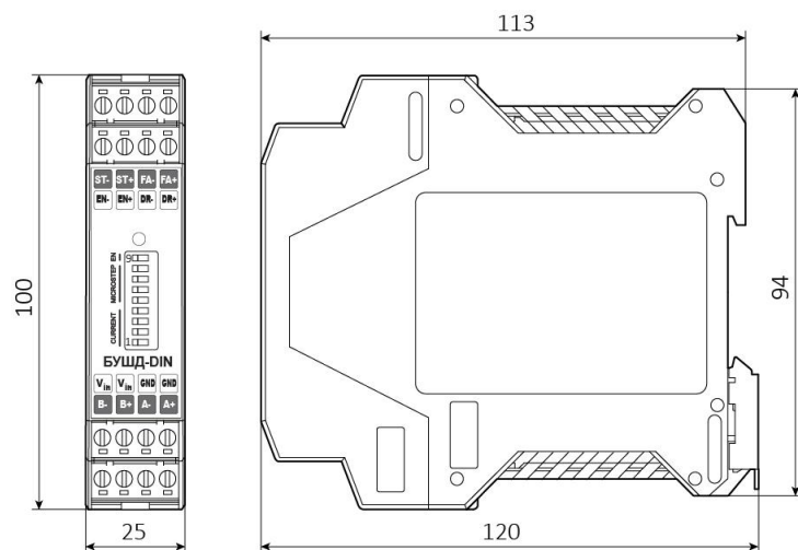
Рис. 6. – Габаритные и присоединительные размеры.
