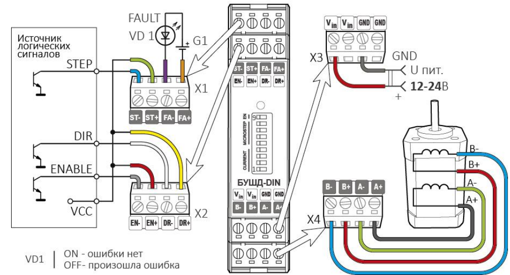
Рис. 1. – Подключение блока по схеме с общим анодом
