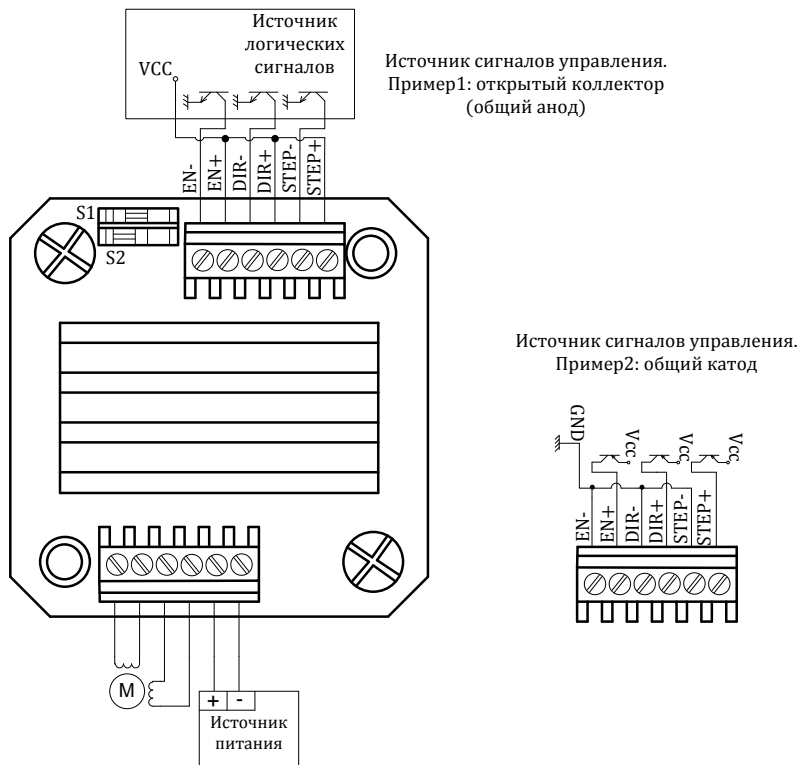
Рис. 3. Схема подключения блока управления SMD-2.8 mini.
