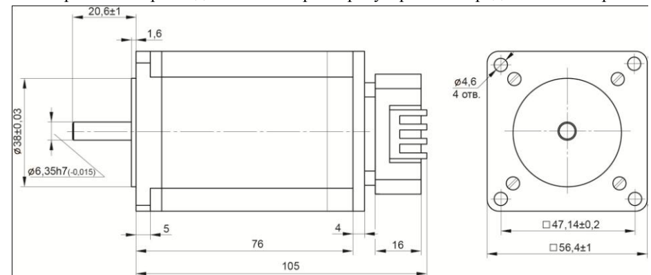
Рис. 2. Габаритные размеры и присоединительные размеры устройства
