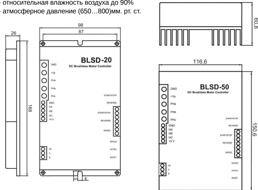
Рис. 1. Габаритные и присоединительные размеры блока BLSД
